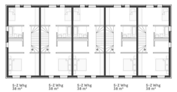
GRUNDRISS 2.OG
